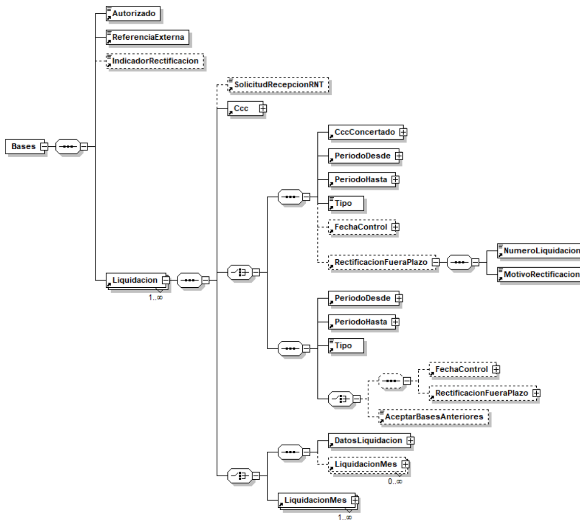
Ilustración 1: Tipo de Dato Bases
